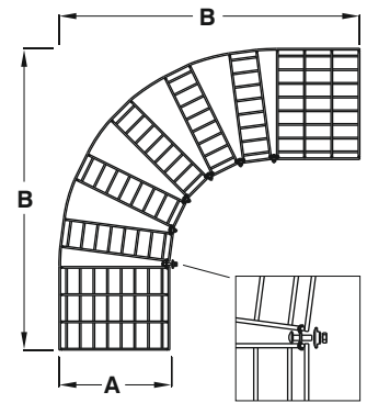
Элемент наращивания длины проволочного кабельного лотка
