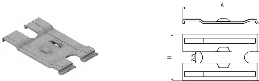
Нижний элемент наращивания длины проволочного кабельного лотка для безболтового соединения
