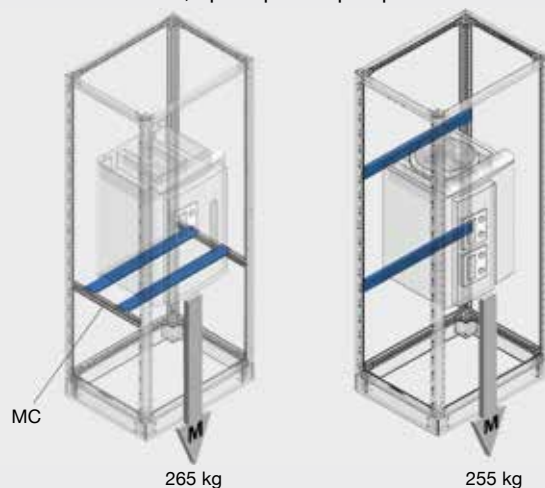
SP, примеры сборки рейки
